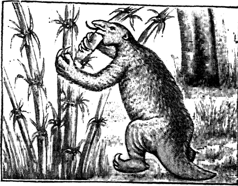
चित्र २०—भीमकाय डिनोसौर
